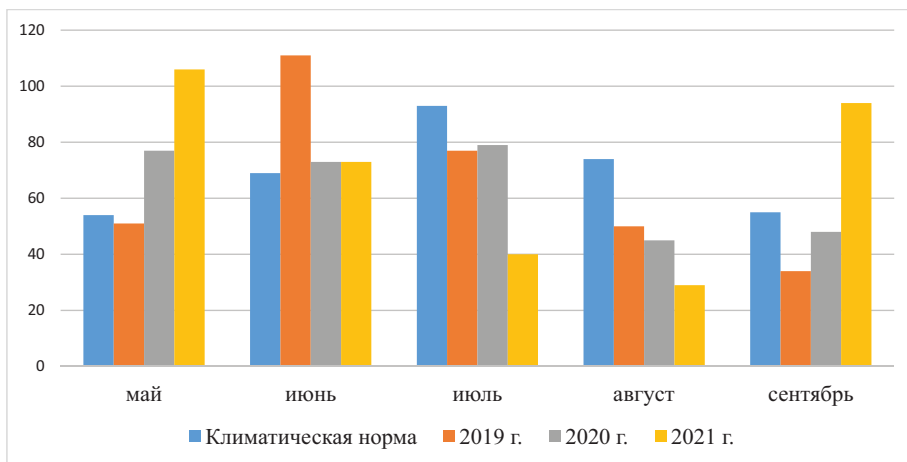
Рис. 2. Количество осадков в вегетационные периоды, мм, г. Калуга, 2019–2021 гг.
