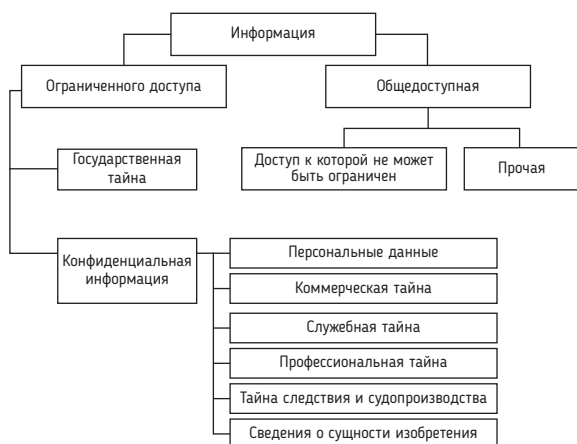
Рис. 1. Виды информации
